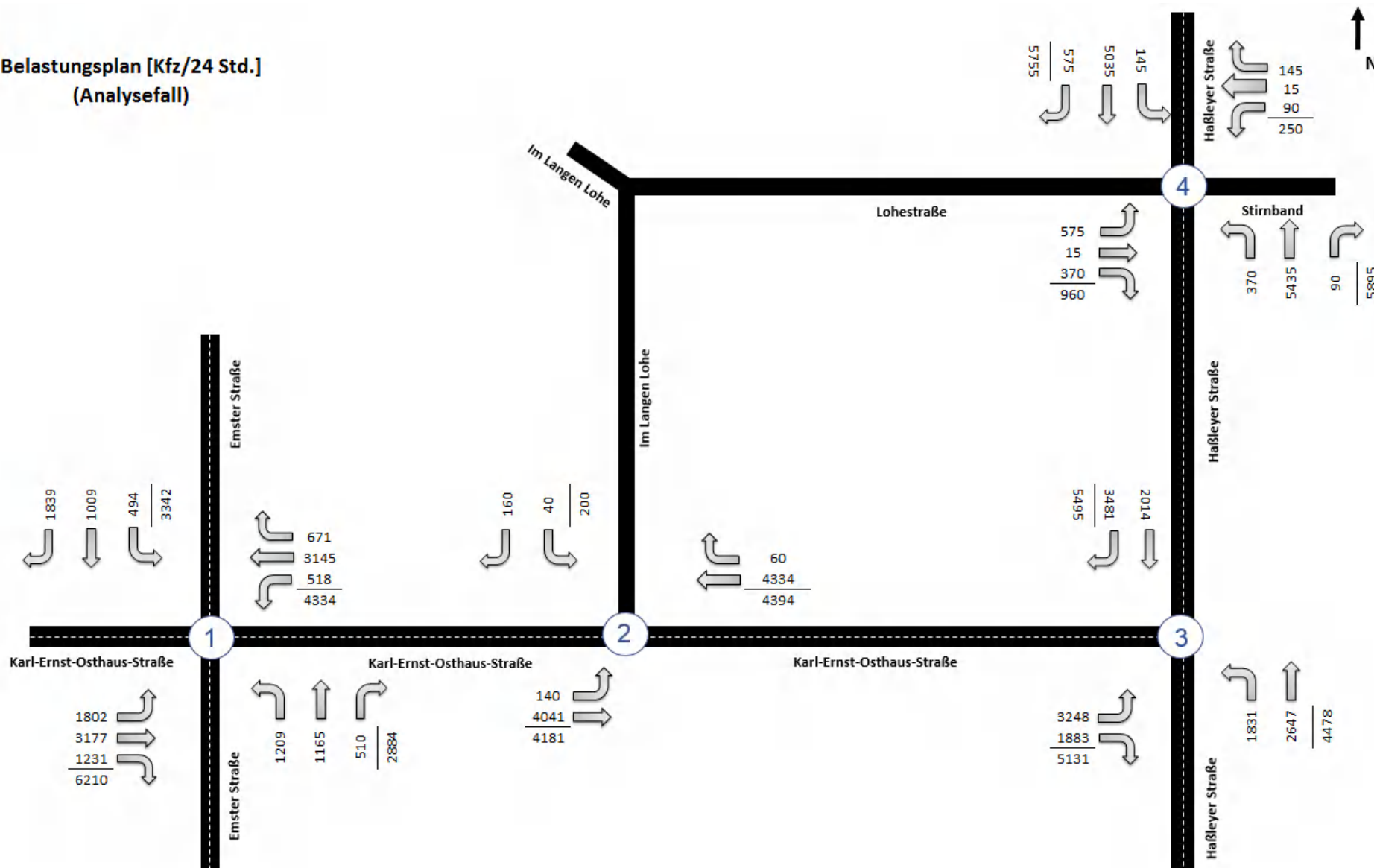
Abbildung 4: Gesamtverkehrsbelastung in 24 Std.
