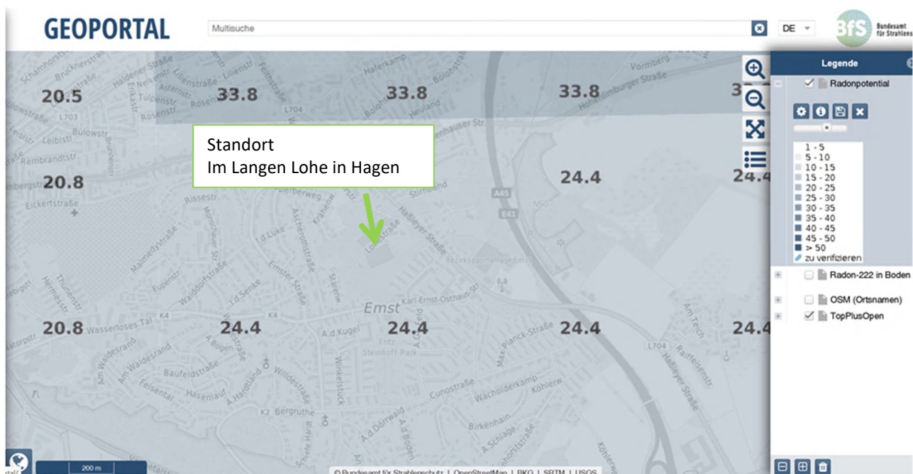
Detailkarte Radonprognose aus dem Geoportal des Bundesamtes für Strahlenschutz (BfS)
