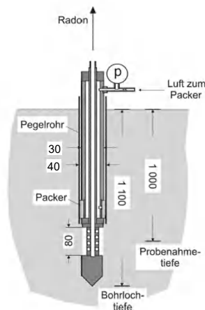
Abb. 1: Packer-Bodengassonde
