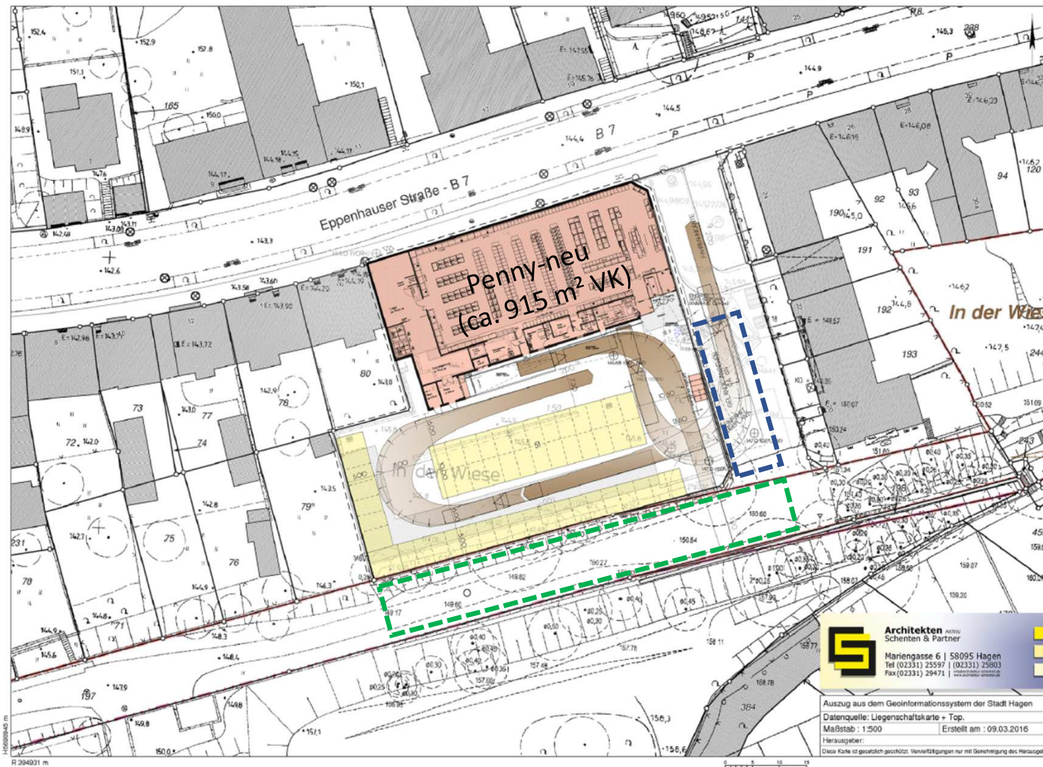
Anlage 1) neuer Penny-Markt inkl. ebenerdiger Stellplatzanlage und erweiterter Erschließung (EG)
