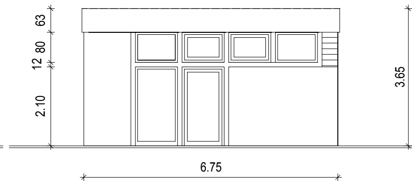
ANSICHT SÜD
