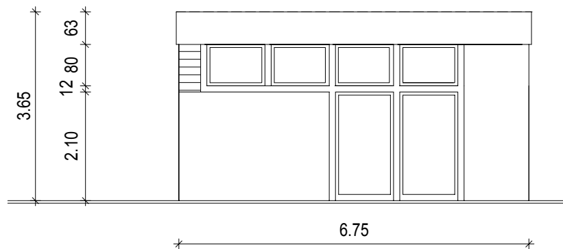
ANSICHT NORD
