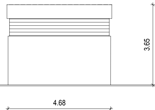
ANSICHT OST
