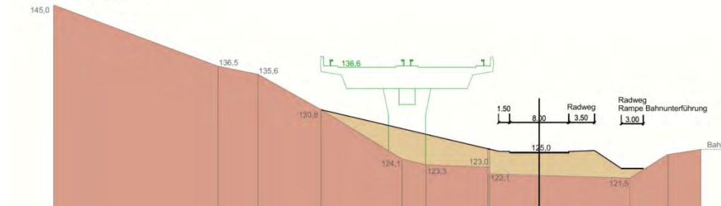
Schnitt G-G
