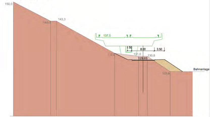
Schnitt F-F
