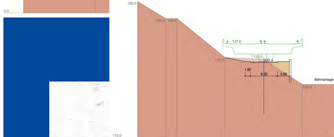
Schnitt G-G
