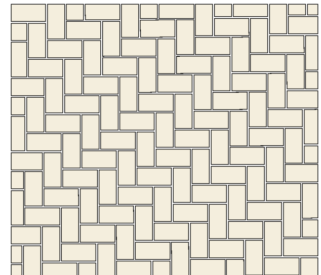
Pflaster Typ Fahrbahn
