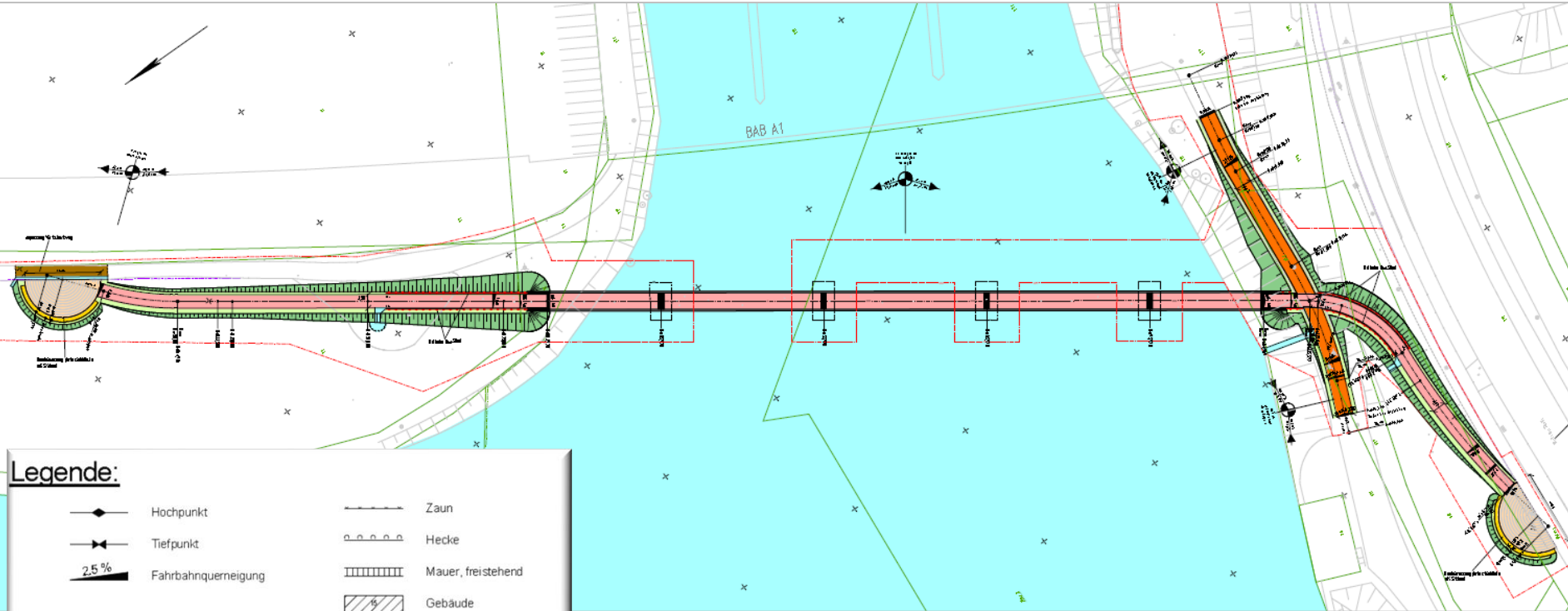
Wegeführung und Aufsicht Brücke
